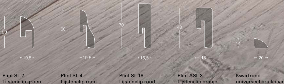
Doorsnede plint
